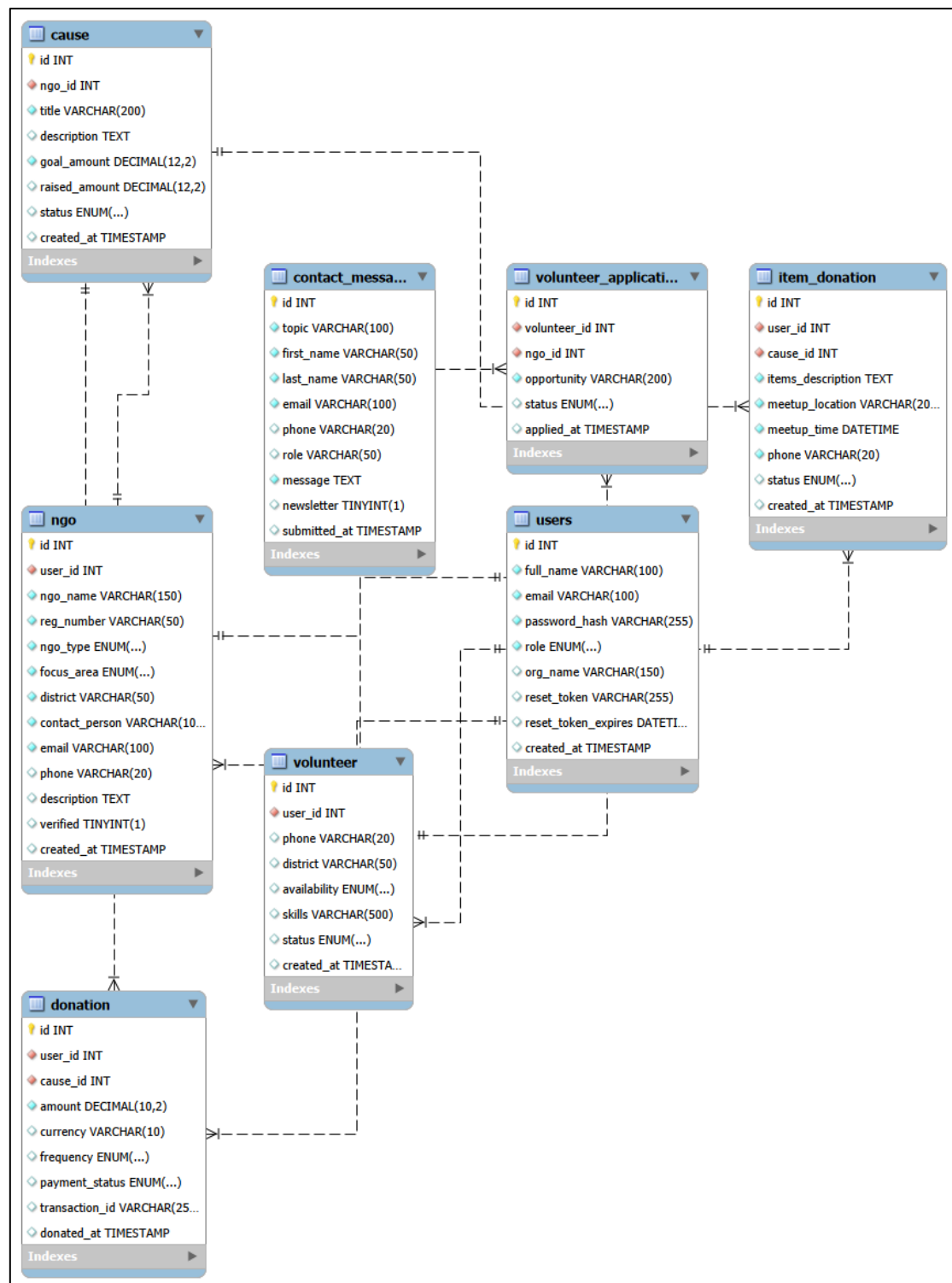
Figure 3: ER Diagram
